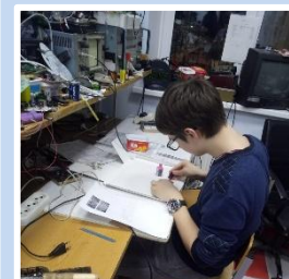
Изготовление печатной платы для схемы
